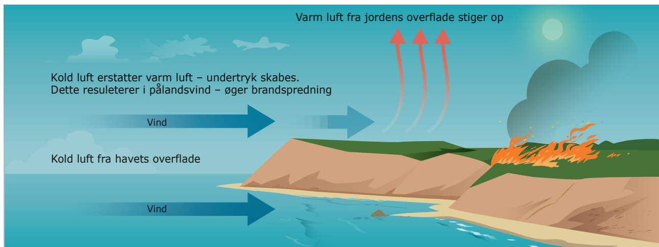
Illustrationen viser havbrisen. Solen har varmet jorden op, så denne er varmere end havets overflade. Når jordens overfladevarme stiger til vejrs, erstattes den af kold luft fra havets overflade. Dette betyder, at der nu opstår en pålandsvind. Denne vind kan påvirke brandforløbet og øge brandspredning Grundet forøget vind. Dette sker oftest i dagtimerne.
