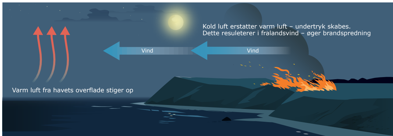
Illustrationen viser landbrisen. Jordens overflade er nedkølet, da solen ikke længere varmer jorden. Nu er jorden koldere end havoverfladen. Der sker nu den modsatte effekt som ved havbrisen. Dette betyder, at der nu opstår en fralandsvind. Denne vind kan påvirke brandforløbet og øge brandspredning, men kan også resultere i det modsatte, da vinde kan presse branden mod et allerede afbrændt område med mulighed for effektiv bekæmpelse. Dette sker oftest i nattetimerne.
