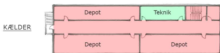
Figur 3: Et eksempel på et daginstitutionsafsnit til flere end 50 personer samt soverumsafsnit med flere end 10 sovepladser. Soverumsafsnittet til højre, som er til højst 10 personer, har ikke fælles flugtveje med de andre soverumsafsnit, hvorfor det skal ansues som et selvstændigt soverumsafsnit, der på grund af personbelastningen ikke er et brandsynsobjekt i sig selv, men det kan undtagelsesvist inddrages i brandsynet af de andre soverumsafsnit, som er indrettet med flere end 10 sovepladser, hvis det konkret skønnes nødvendigt for at forebygge eller mindske brandfaren, og for at sikre forsvarlige rednings- og slukningsmuligheder i tilfælde af brand, jf. § 2, stk. 7, i bekendtgørelsen. Brandsynet omfatter bygningens stueplan. I kælderen omfatter brandsynet teknikrummet, idet der i det konkrete tilfælde er tale om et ventilationsrum, som via ventilationskanaler er i direkte tilknytning med daginstitutionsafsnittet og soverumsafsnittene i stueplan. De øvrige rum i kælderen er ikke opholdsrum, og har ikke direkte tilknytning til brandsynsobjekterne i stueplan.
